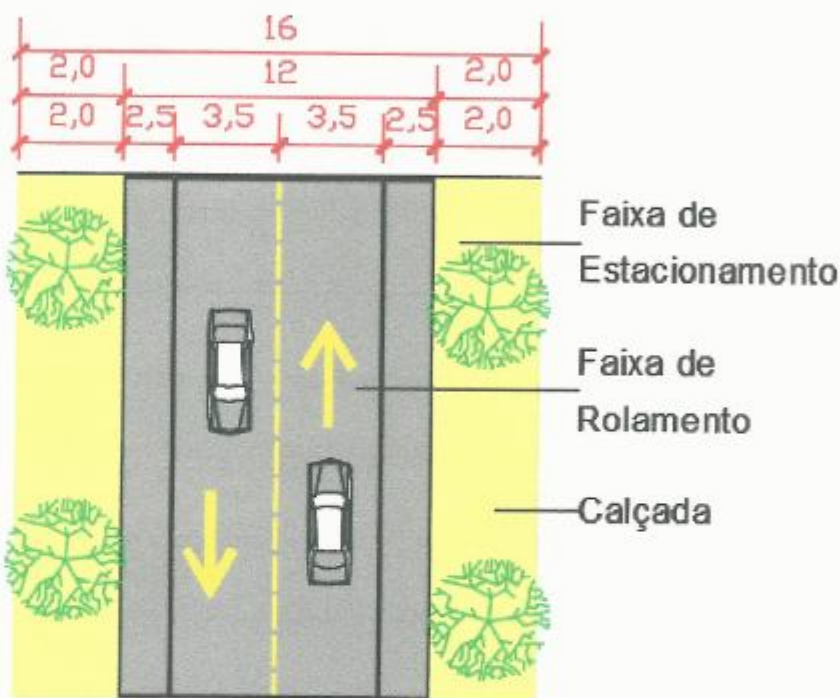
Planta Esquemática
